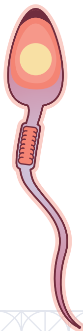
SPERMATOZOÏDE
