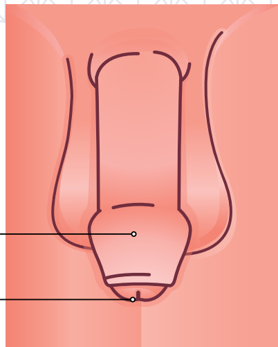
PÉNIS
