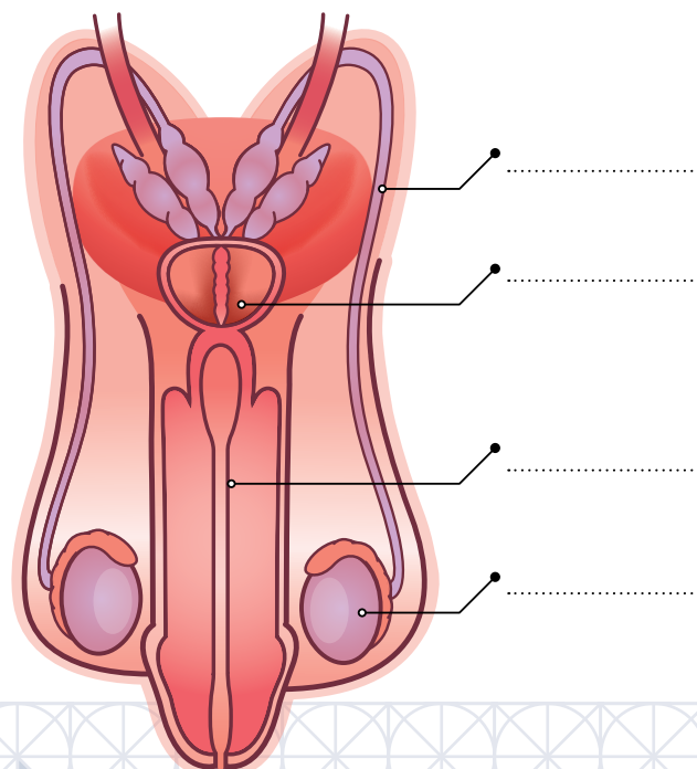
PÉNIS
